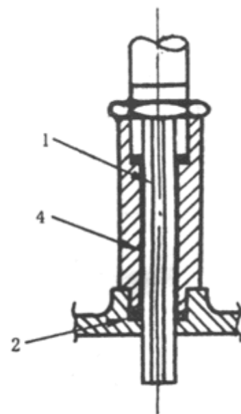
导管引入装置
