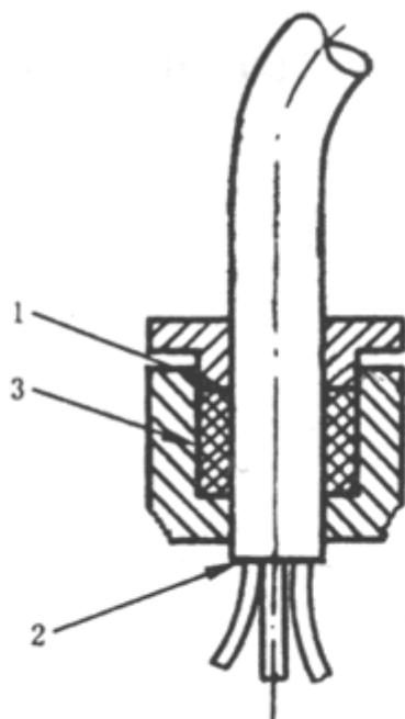
电缆引入装置
